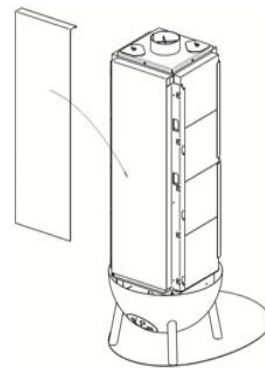
Lämpösuoja taakse palosuojaetäisyyden pienentämiseen
