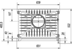
Топка для камина ZUZIA 16 кВт
